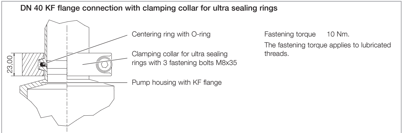
Abb. 3.5 Hochvakuumflansch DN 40 KF befestigen
