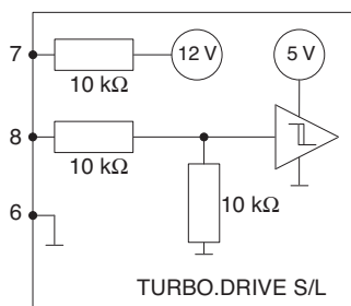
Abb. 4 Belegung der Gerätebuchse REMOTE IN
